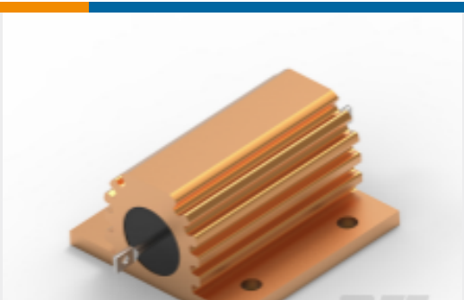
TE 产品编号5-1630186-7 功率电阻器：铝壳体，HSA
