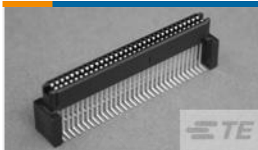
TE 产品编号2007042-4 1FHR,64,50A/P,S,C,R14,15
