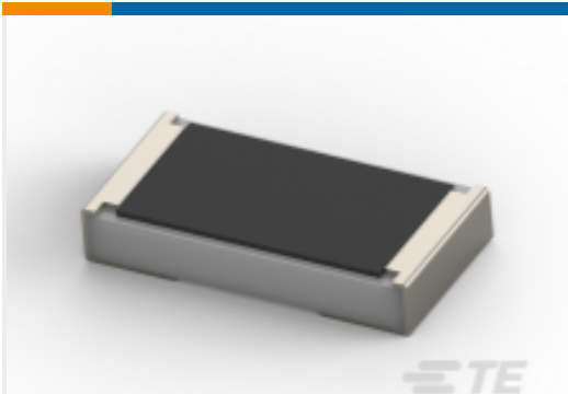
TE 产品编号2-2176232-1 SMD 功率电阻器：3 瓦特，1% Tol
