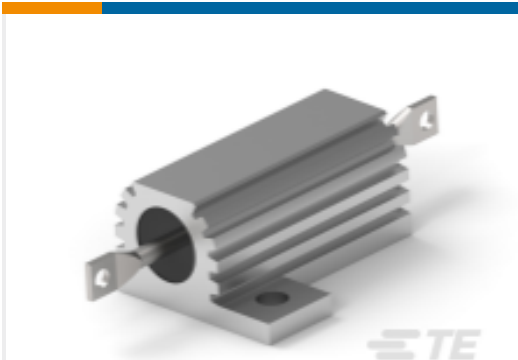
TE 产品编号1-1879074-1 功率电阻器：铝壳体，75 瓦特
