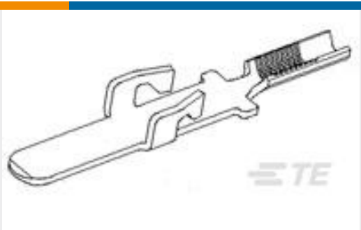
TE 产品编号1217072-1 CONT AMVAR 125 BLADE 020 TPBR
