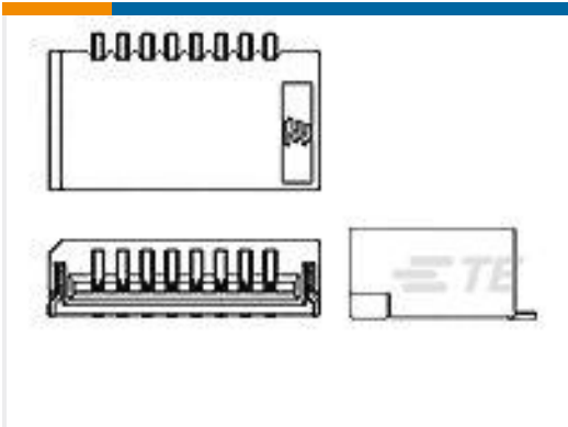
TE 产品编号1-84981-0 1MM FFC SMT H ASSY 10P EMBOSS
