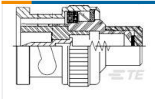
TE 产品编号1-1337523-0 BNC Plg Term 50Ohm Nickel Pltd
