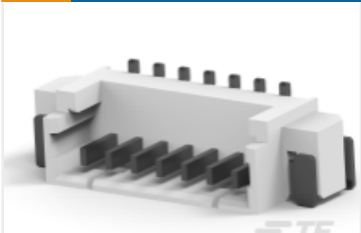
TE 产品编号1734829-2 AMP HPI 1.25MM 接头
