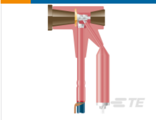
TE 产品编号555340-070 RICS 非绝缘 T 型适配器
