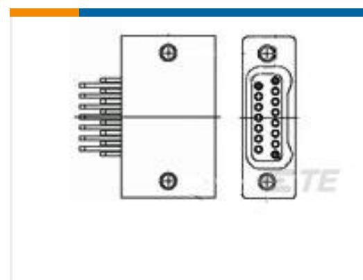
TE 产品编号1-1589483-7 STL025L2HN = SMT CONN
