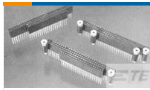
TE 产品编号1375795-4 PC104 ASY STKTHRU UNKEYED LF
