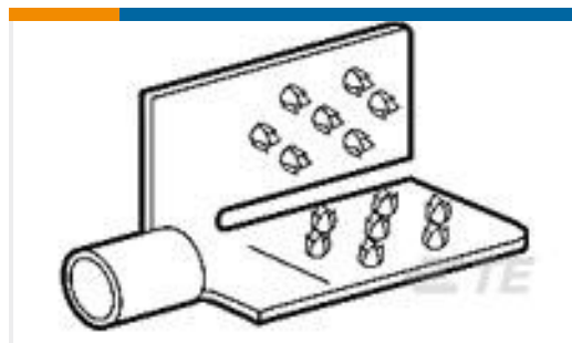
TE 产品编号1-330716-3 TERMINAL,TERMI-FOIL 12-10
