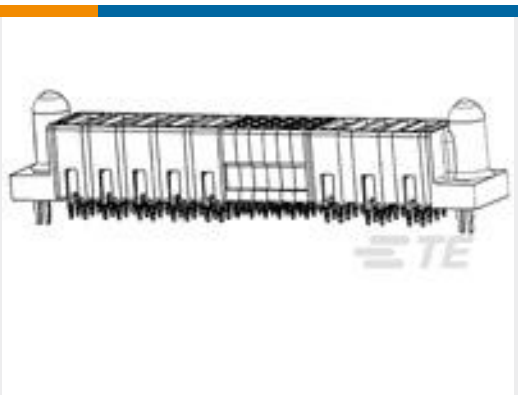
TE 产品编号1892430-5 MBXL VERT RCPT 2P+24S+2P
