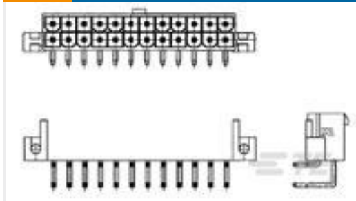
TE 产品编号2-1586043-4 24P VAL-U-LOK R/A HDR SCRMT V2
