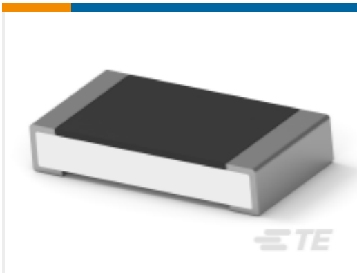
TE 产品编号1-2176391-0 RQ 1206 15K4 0.1% 10PPM 5K RL
