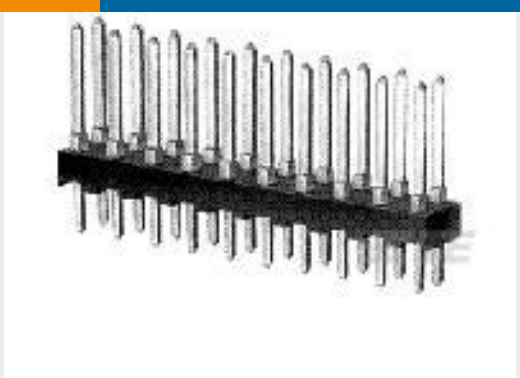
TE 产品编号1-87215-0 02 MODII HDR DRST UNSHRD .100
