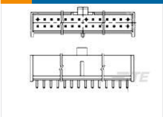
TE 产品编号1-1658549-6 FPH-2022T=FLXPAC HDR P 20 ST LF
