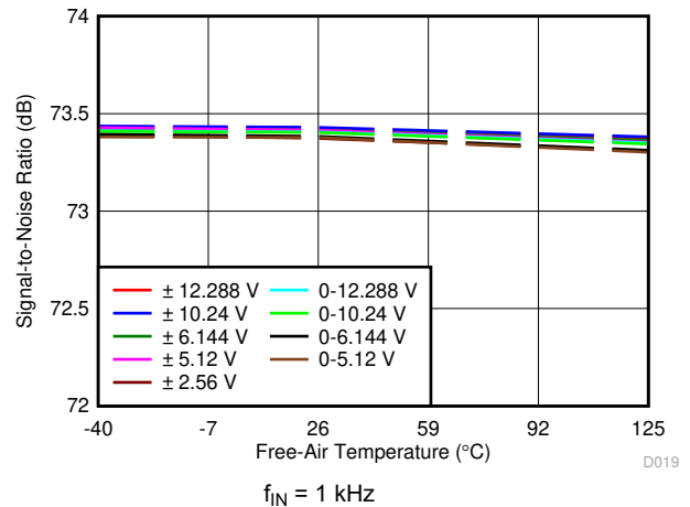
图 6-36. SNR vs Temperature
