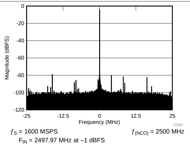
图 111. Spectrum — Decimate-by-32
