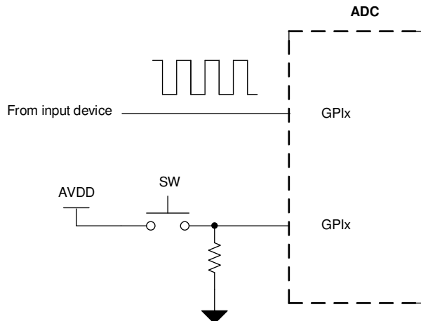
图 150. Digital Input
