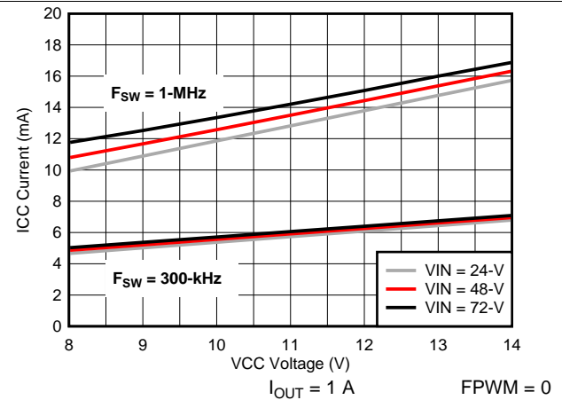
图 8. I_{CC} vs External V_{CC}
