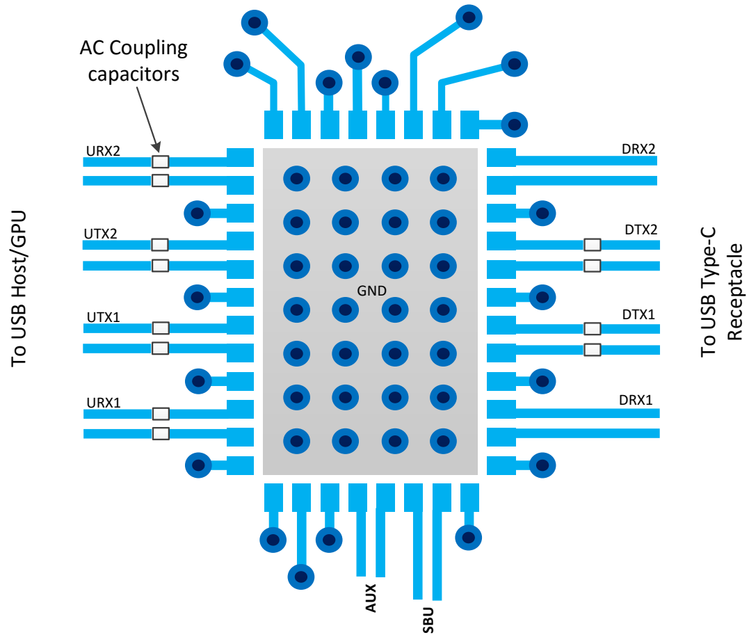
图 52. Example Layout
