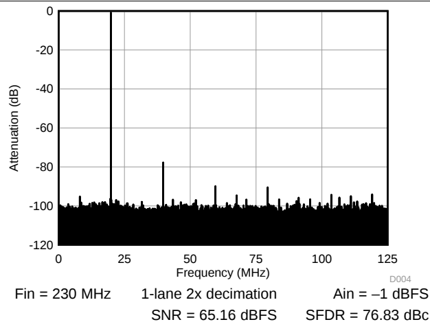
图 8. FFT 230 MHz
