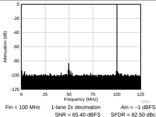
图 6. FFT 100 MHz
