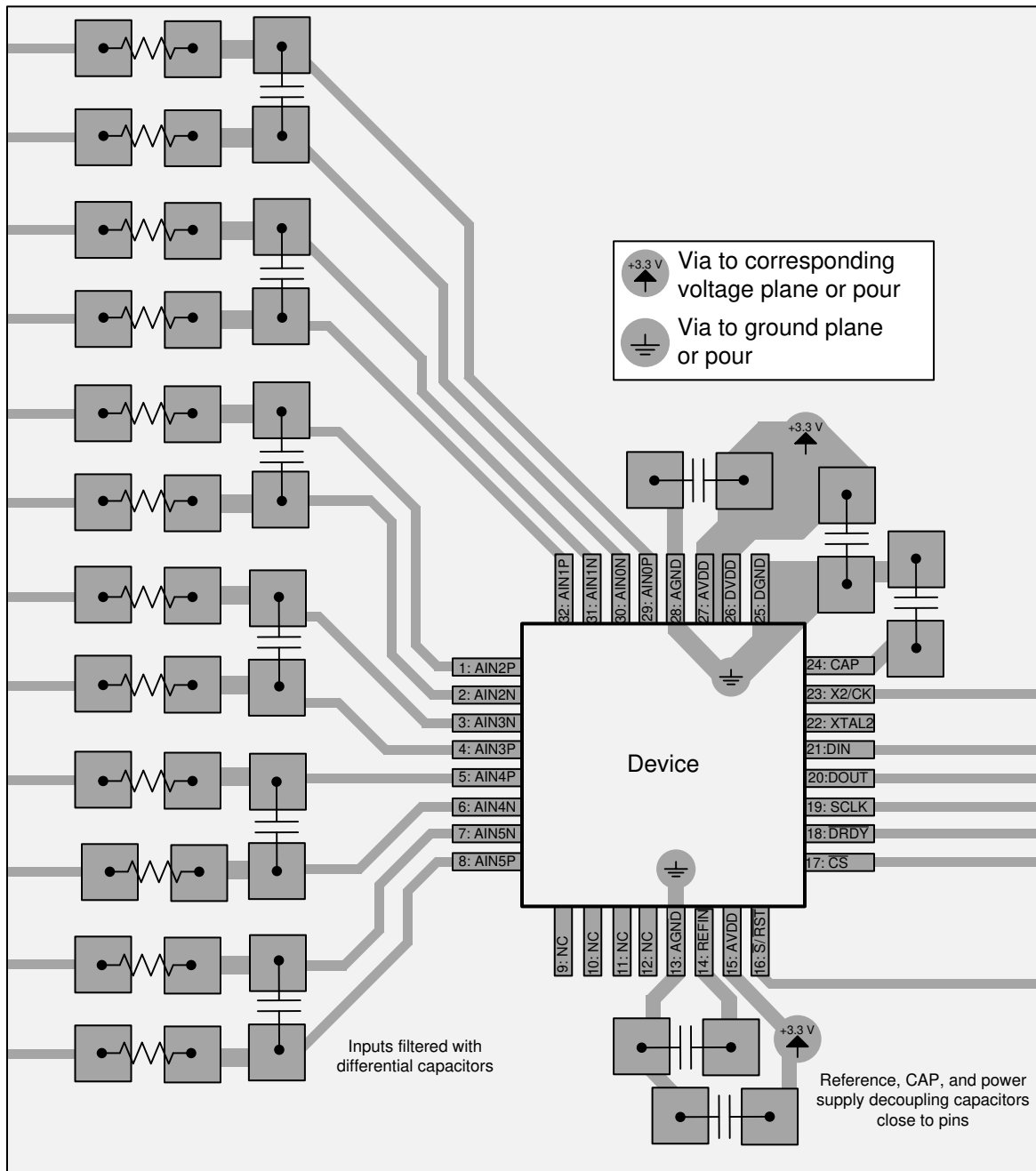
图 98. Layout Example
