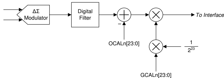
图 36. Calibration Block Diagram
