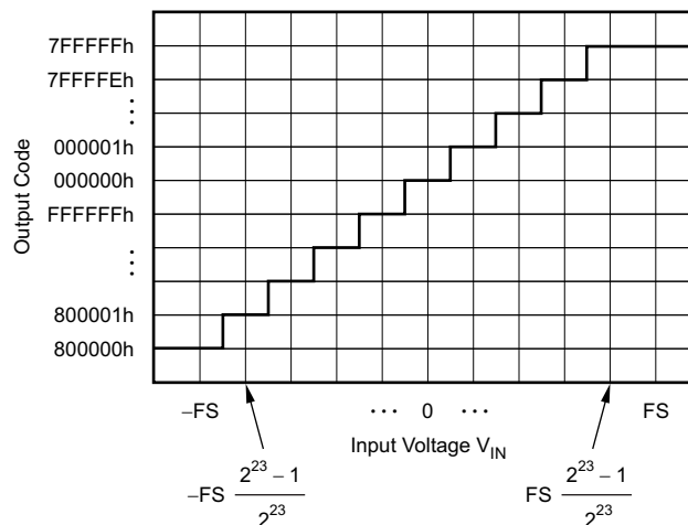
图 41. Code Transition Diagram
