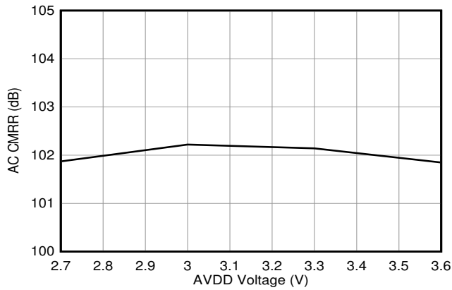
图 16. AC CMRR vs AVDD
