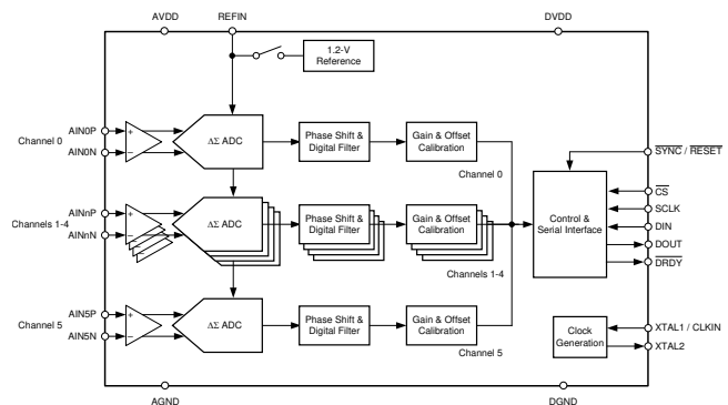
简化方框图
