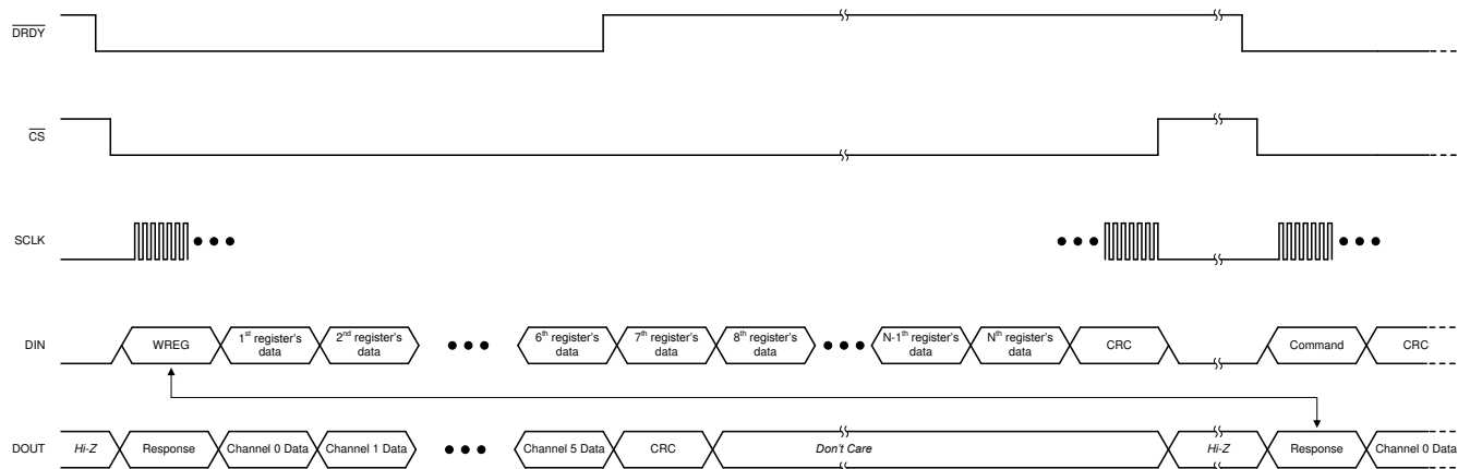
图 47. Writing Registers
