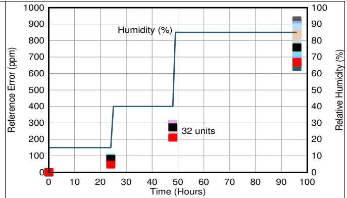
图 23. Reference Error vs Humidity
