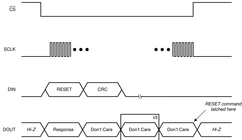
图 44. RESET Command Frame
