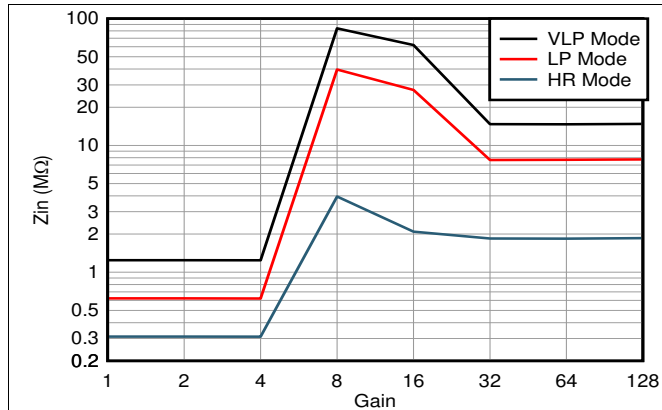
图 4. Input Impedance vs Gain
