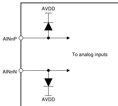
图 24. Input ESD Protection Circuitry
