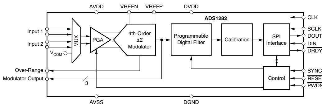
简化原理图
