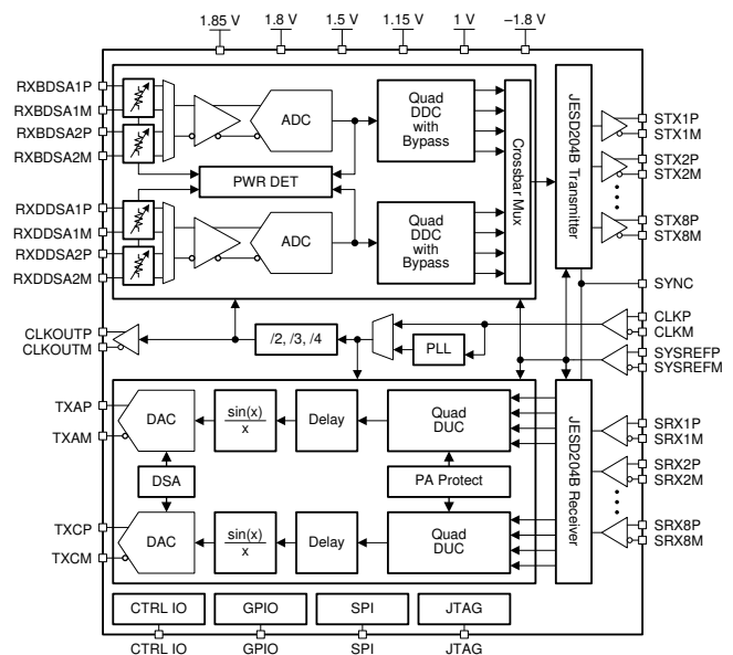
功能框图
