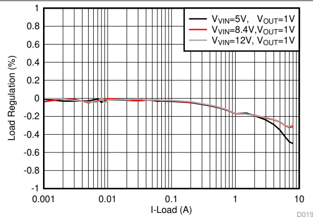
图 32. Load Regulation
