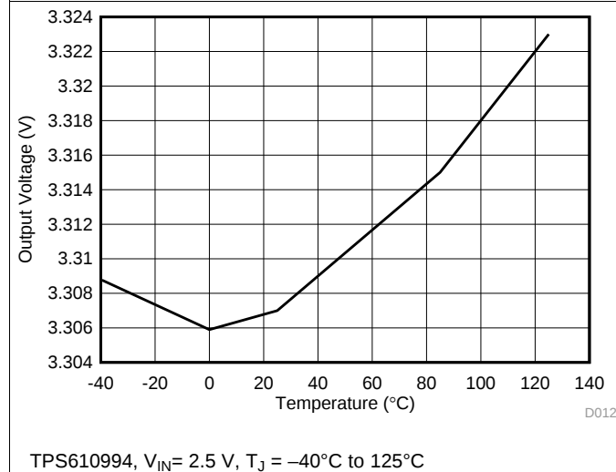
图 15. TPS610994 Output Voltage vs Temperature
