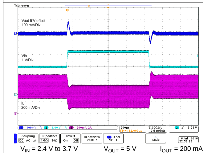
图 25. Line Transient
