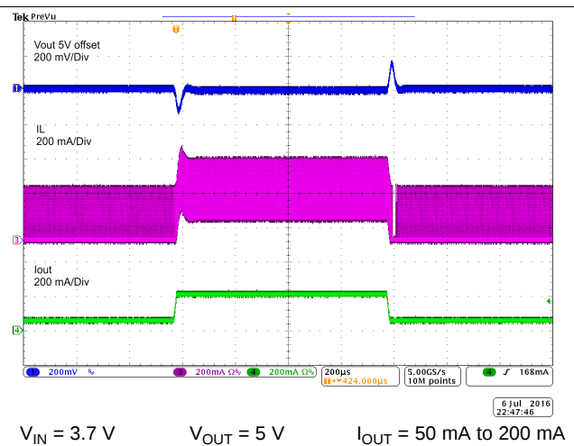
图 26. Load Transient
