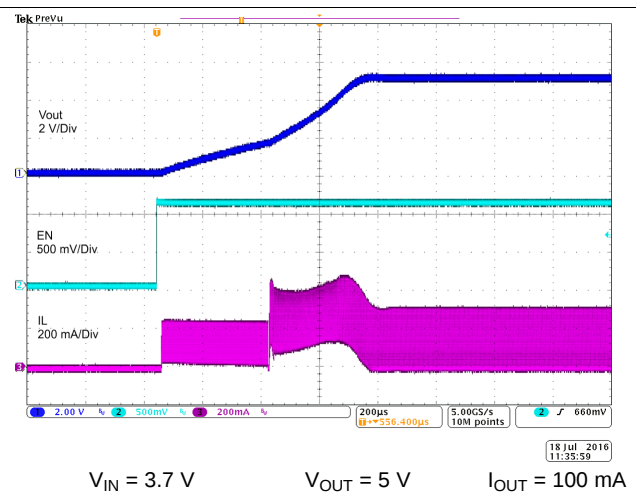
图 24. Startup by EN
