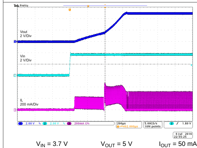
图 23. Startup by V_{IN}
