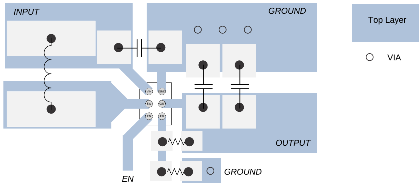
图 29. Layout -YFF
