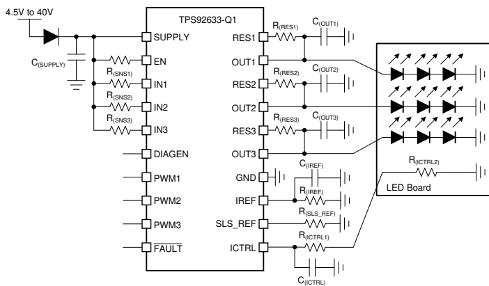
典型应用图
