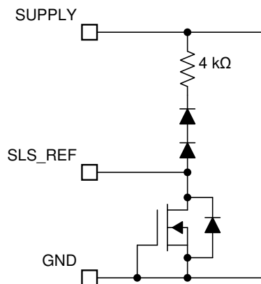
图 7-23. SLS_REF Pin
