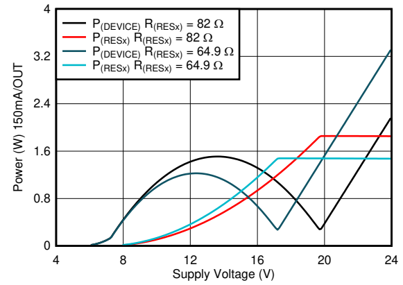
器件功耗
