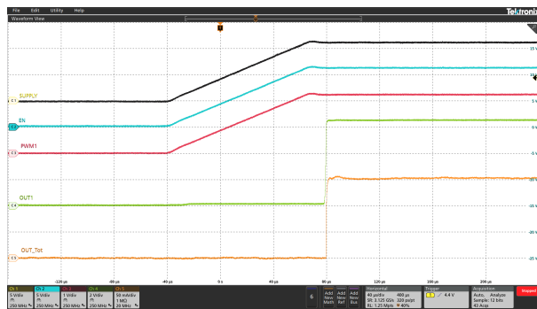
图 6-7. Power Up Sequence
