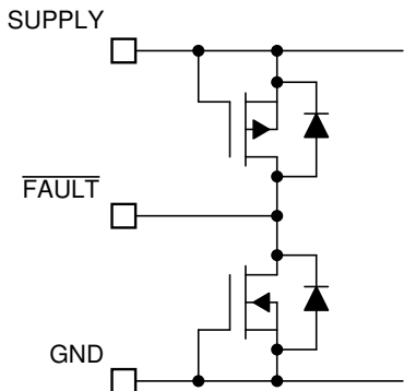
图 7-17. FAULT Pin
