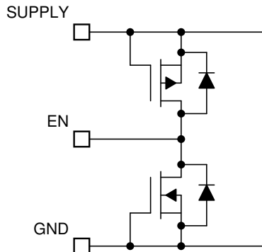
图 7-14. EN Pin
