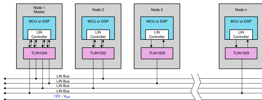
简化原理图
