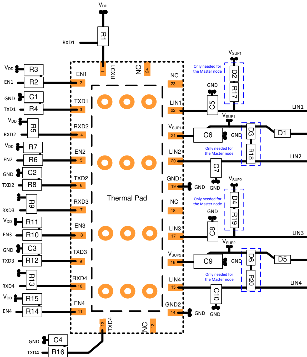
图 33. Layout Example
