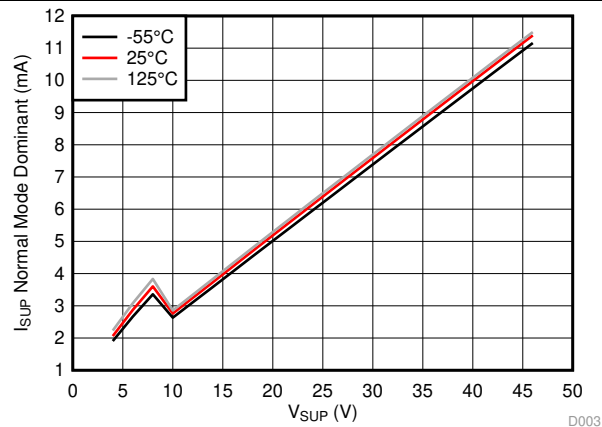
图 3. Normal Mode Dominant vs V_{SUP}
