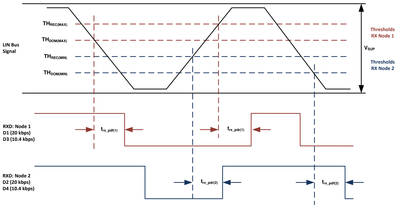
图 21. Propagation Delay
