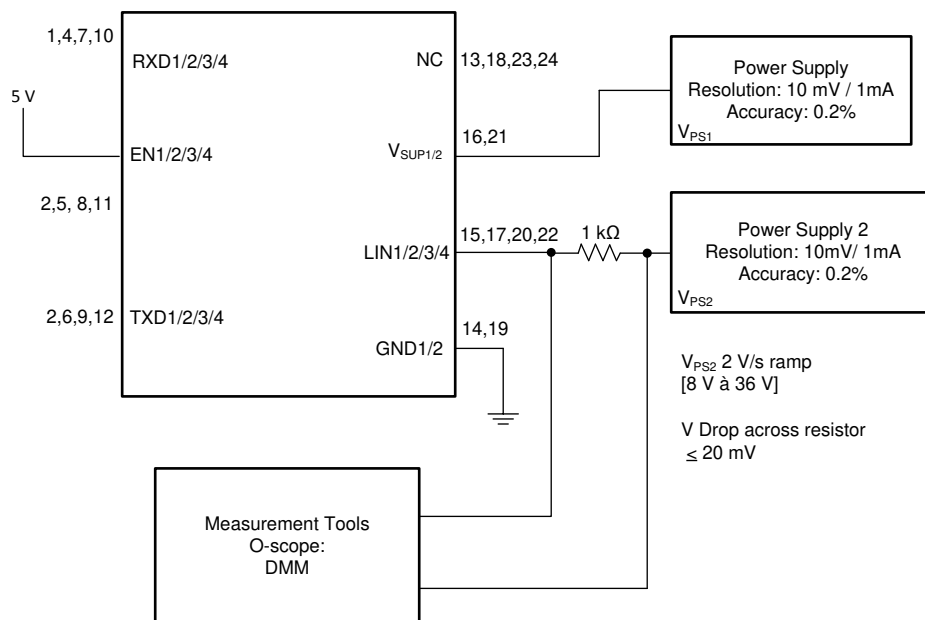
图 15. Test Circuit for I_{BUS\_PAS\_rec}
