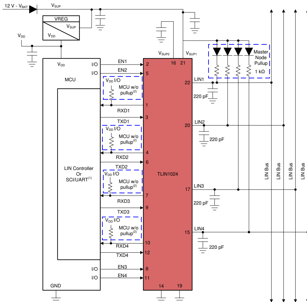
图 30. Typical LIN Bus
