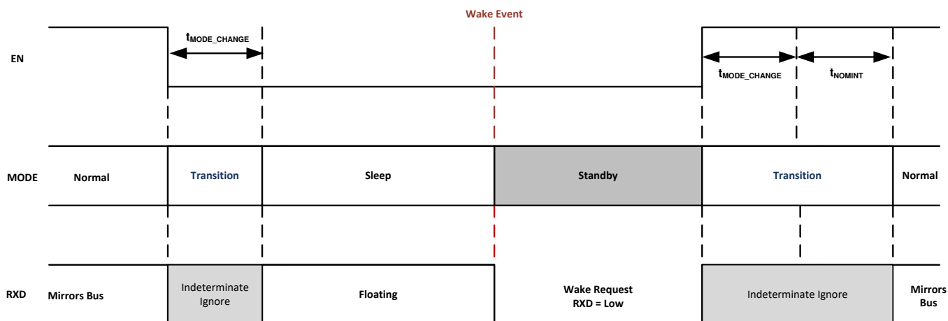
图 22. Mode Transitions
