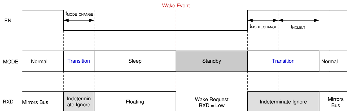
图 7-15. Mode Transitions
