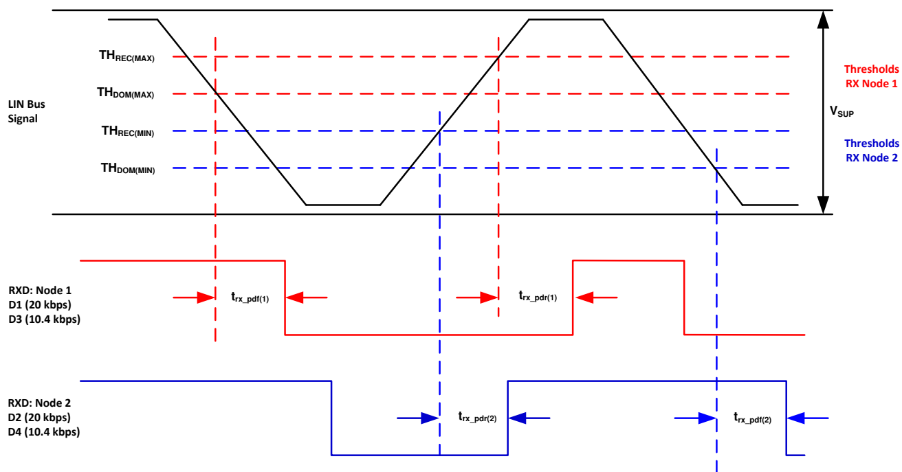
图 7-14. Propagation Delay
