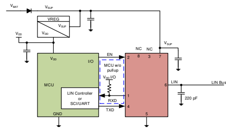
简化版原理图，跟随者模式 (2)
