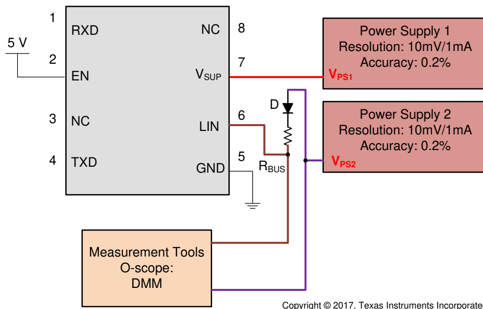
图 7-5. V<sub>SUP</sub>_NON_OP Param 11
