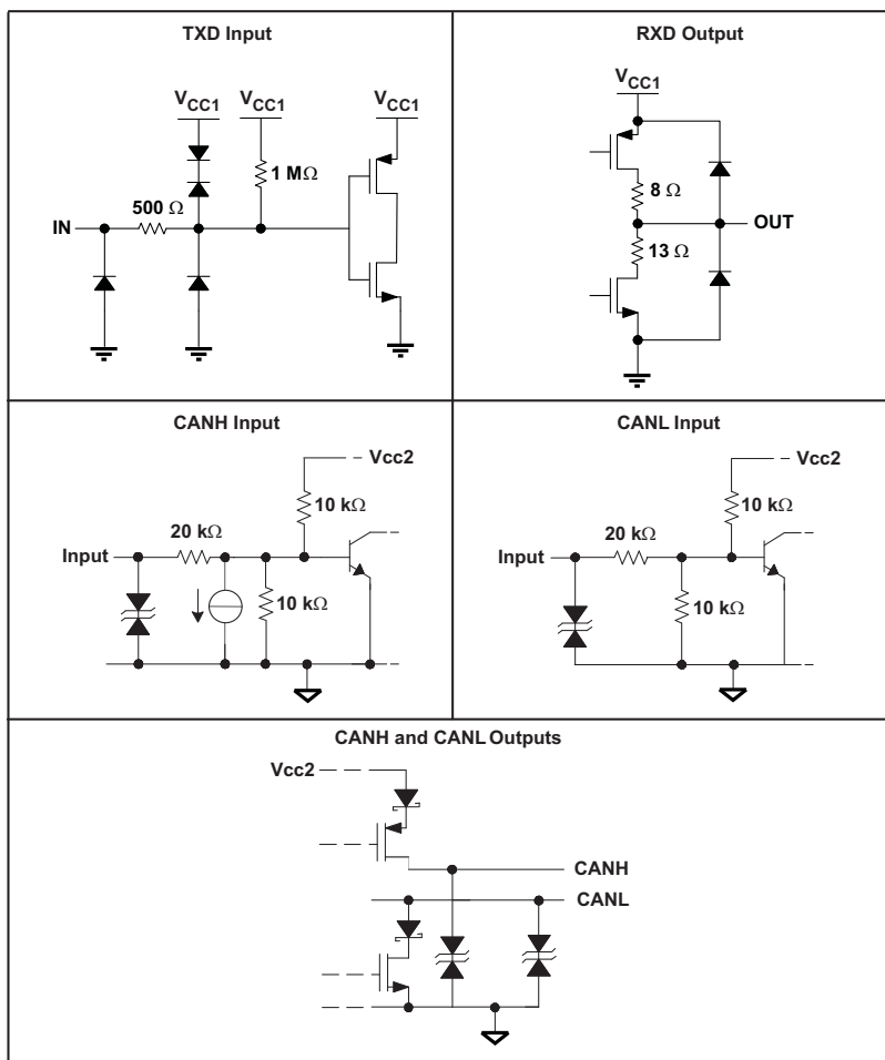
图 26. Equivalent I/O Schematics
