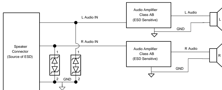
典型应用电路原理图
