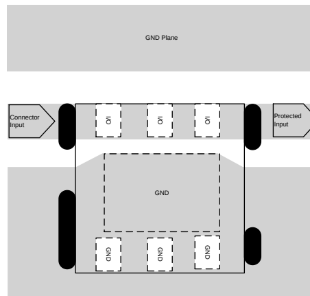
图 12. TVS2200 Layout
