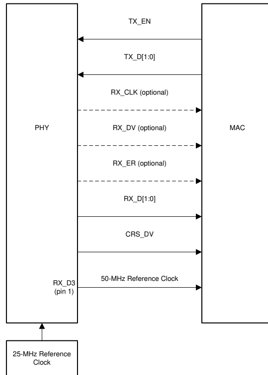
图 13. RMII Master Signaling
