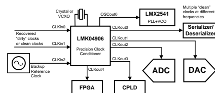
简化 LMK04906 方框图
