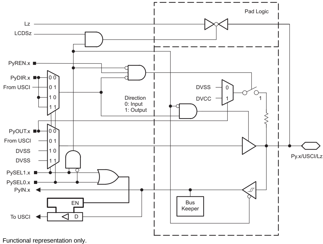
图 6-8. Py.x/USCI/Lz Pin Schematic
