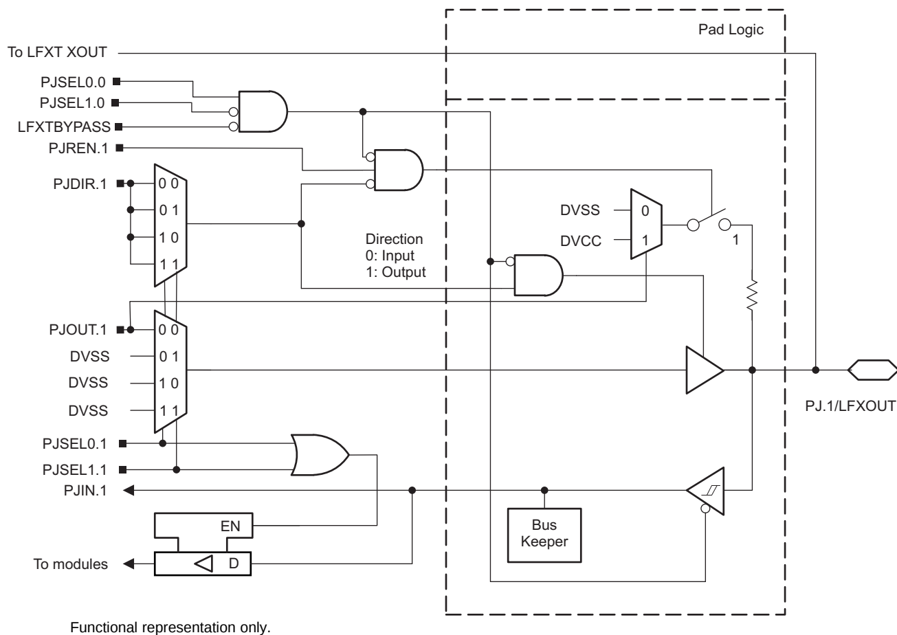
图 6-21. Port PJ (PJ.1) Schematic
