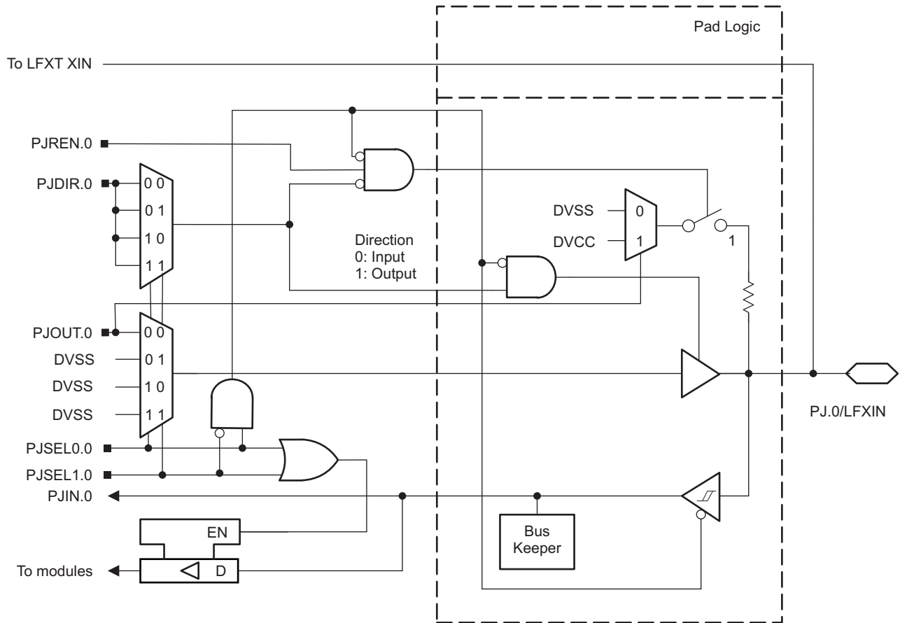
图 6-20. Port PJ (PJ.0) Schematic
