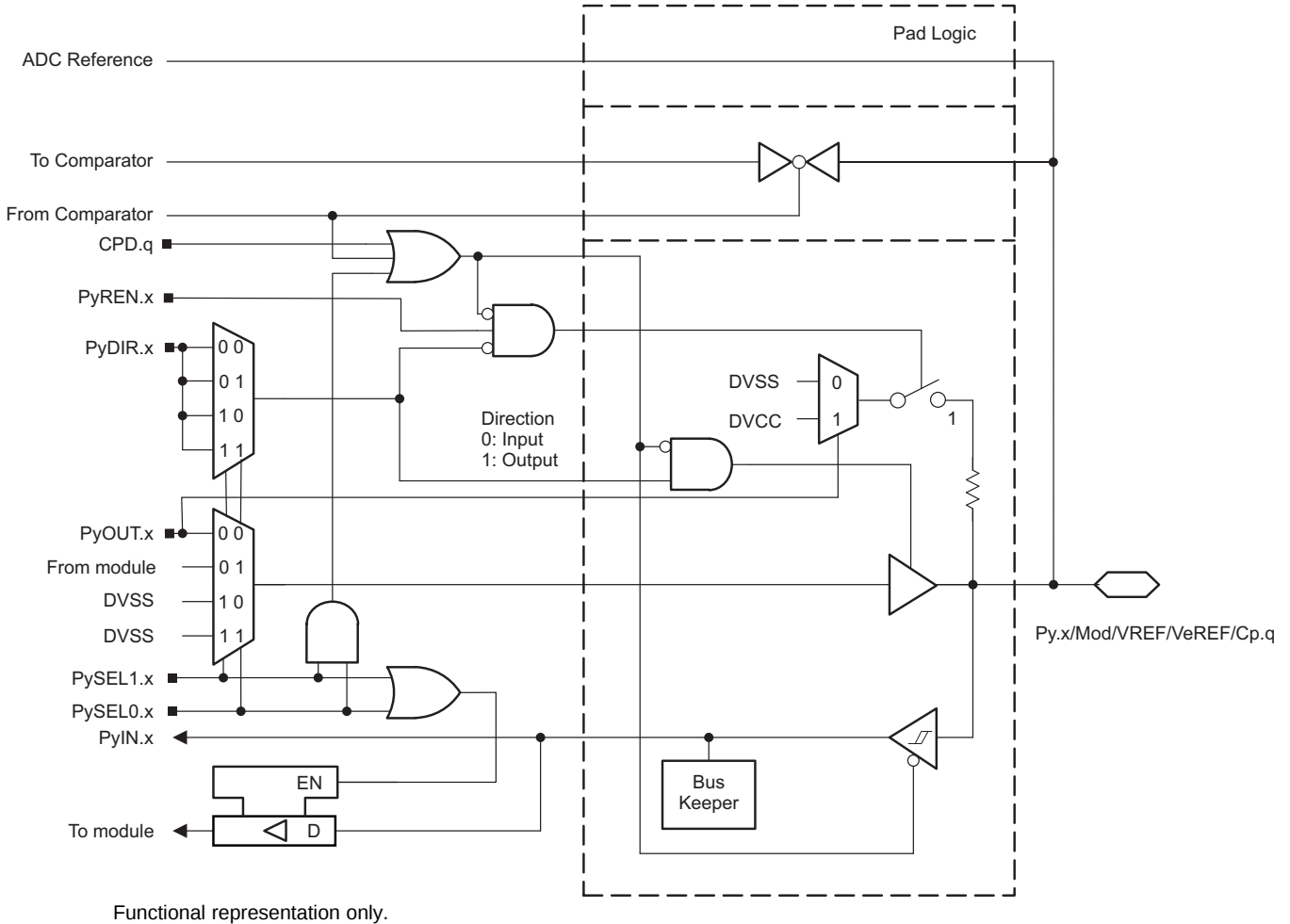
图 6-14. Py.x/Mod/VREF/VeREF/Cp.q Pin Schematic
