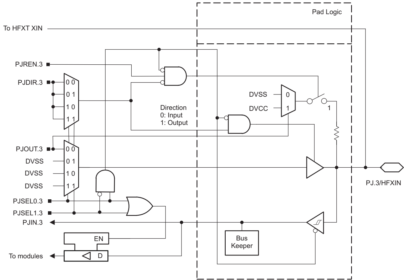
图 6-23. Port PJ (PJ.3) Schematic
