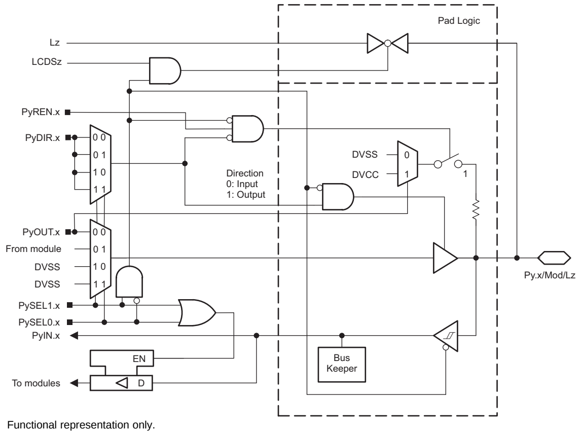
图 6-9. Py.x/Mod/Lz Pin Schematic
