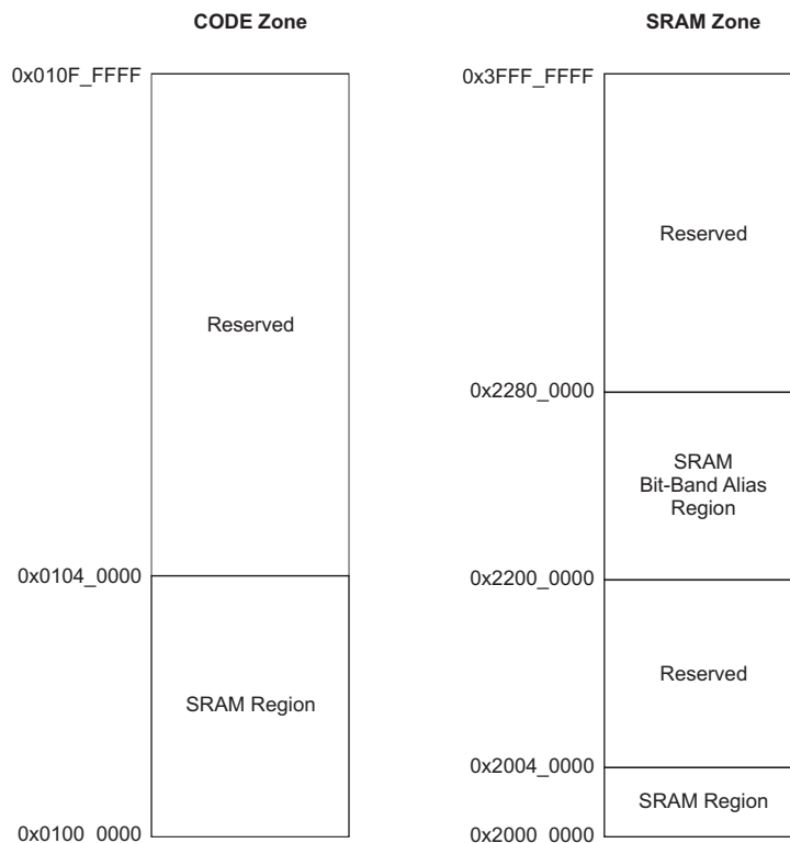
图 6-6. SRAM Map
