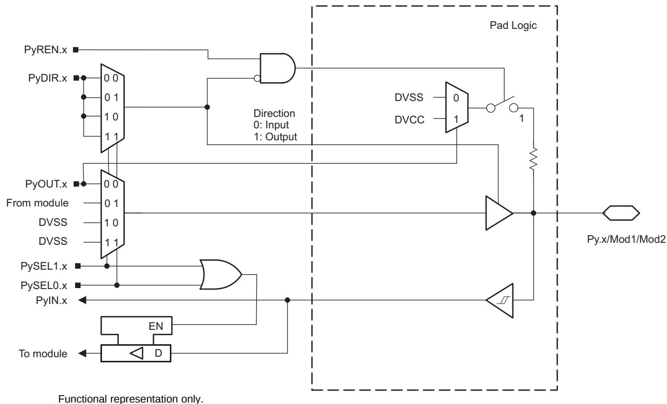
图 6-11. P7.3 Pin Schematic
