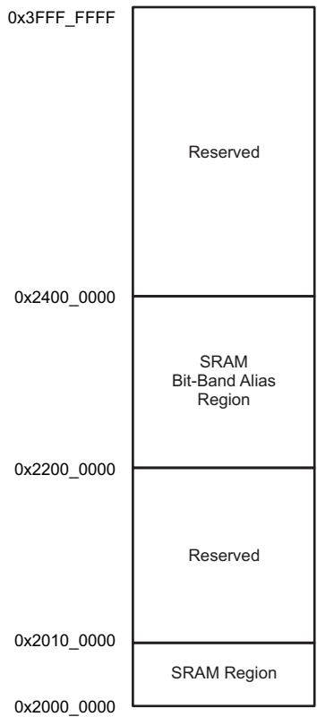
图 6-3. SRAM Zone Memory Map
