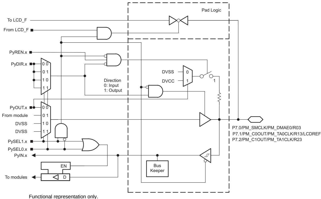
图 6-10. P7.0, P7.1 and P7.2 Pin Schematic
