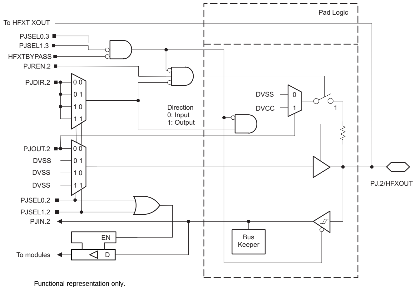
图 6-22. Port PJ (PJ.2) Schematic
