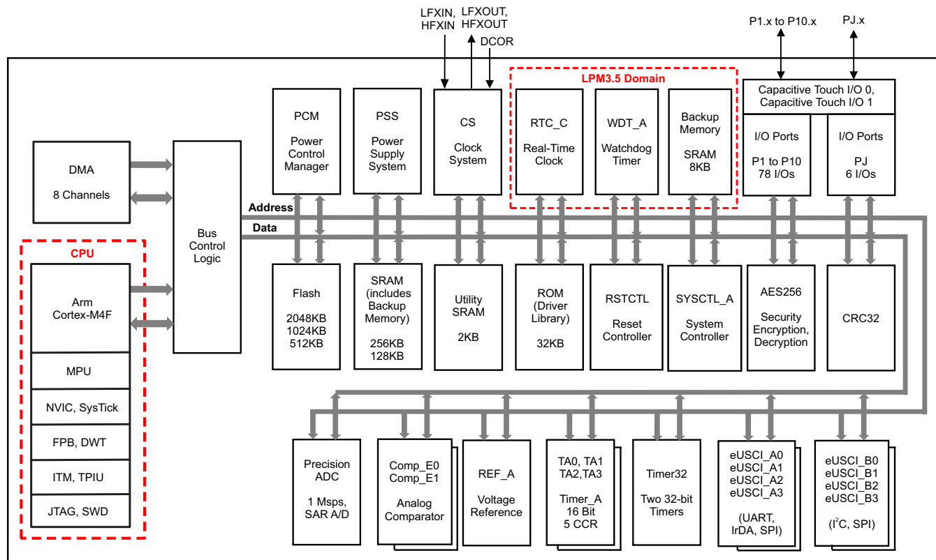
图 1-2. MSP432P401xT 功能框图
