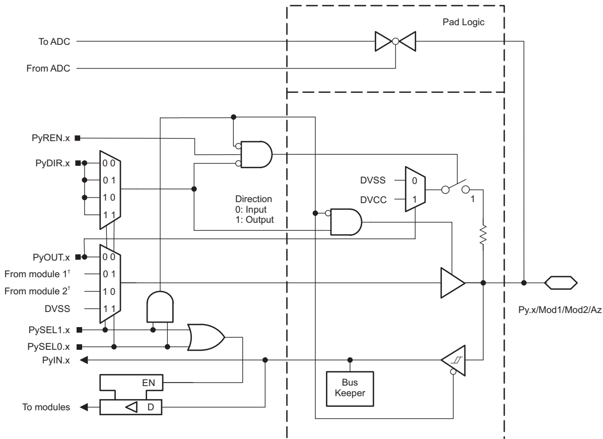
图 6-12. Py.x/Mod1/Mod2/Az Pin Schematic
