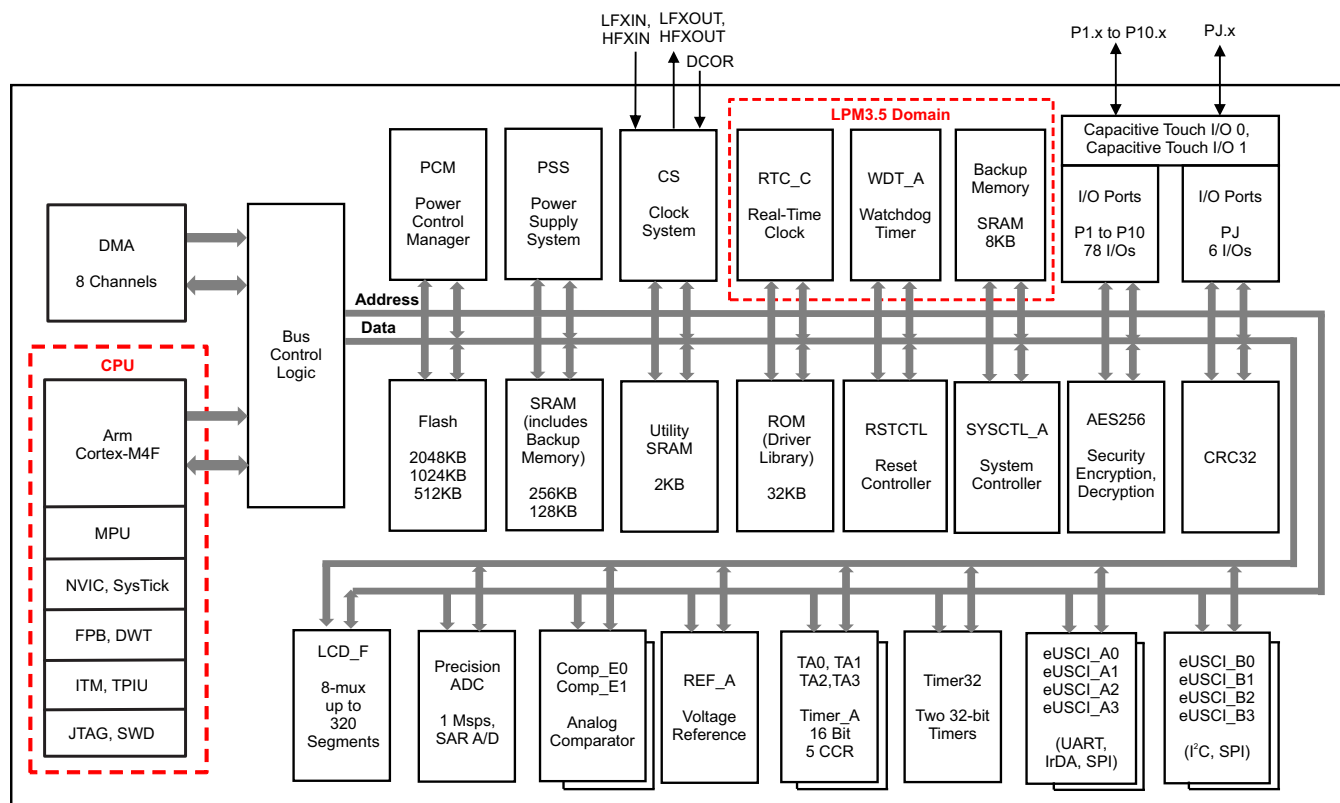
图 1-1. MSP432P411xT 功能框图
