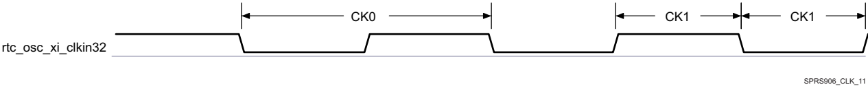
图 6-13. rtc_osc_xi_clkin32 Input Clock
