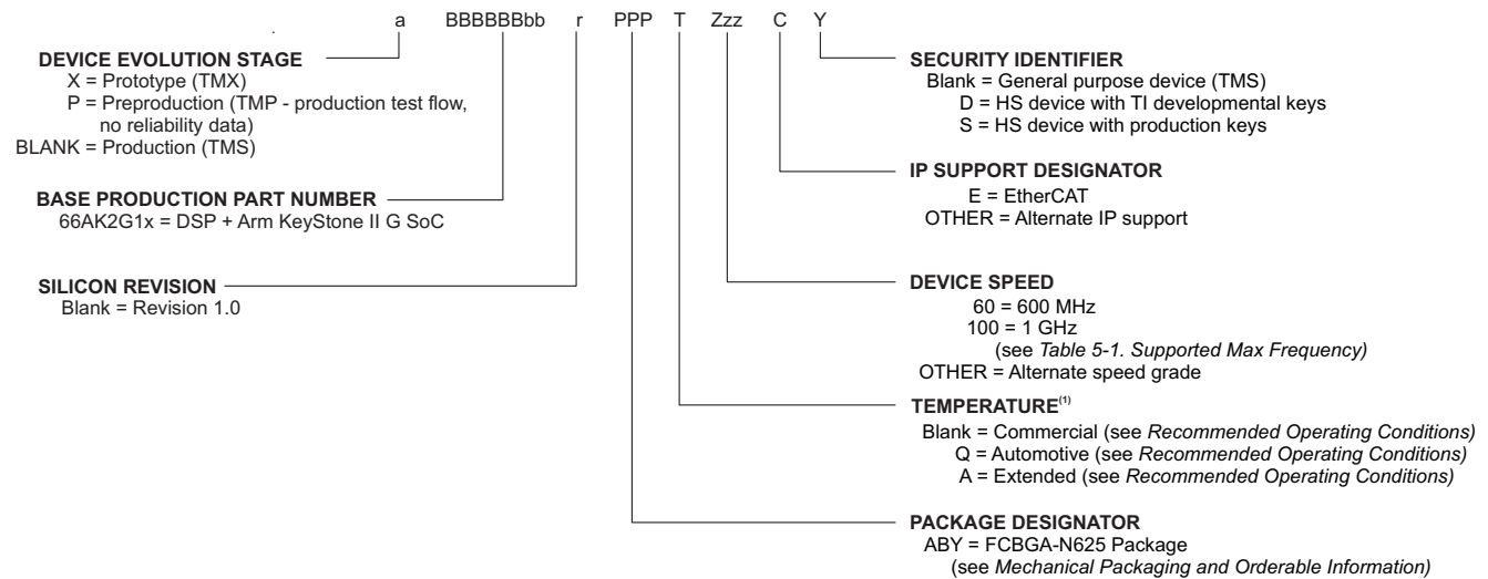
图 8-1. Device Nomenclature
