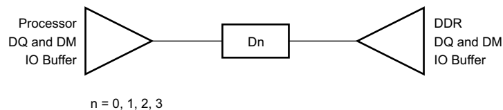
图 7-17. DQ/DM Topology
