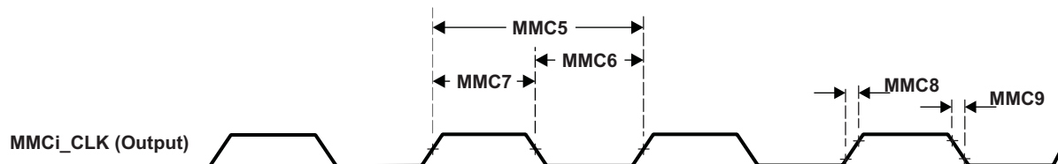
图 5-59. MMCi_CLK Timing (1)
