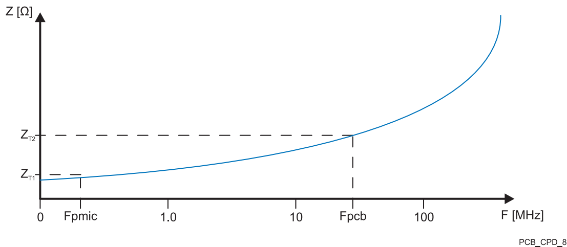
图 8-14. PDN's Target impedance
