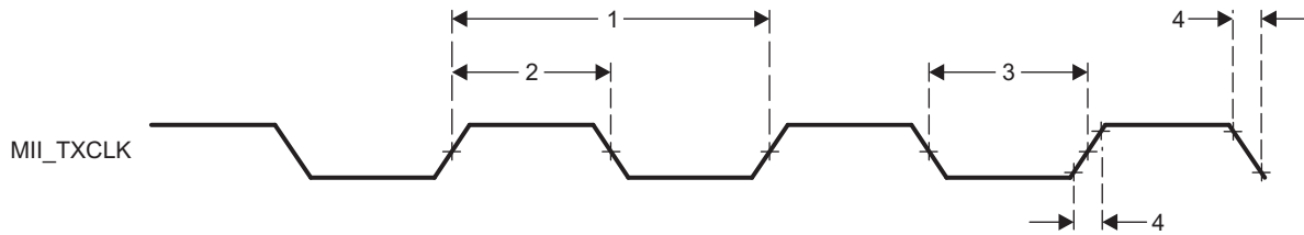
图 7-105. PRU-ICSS MII[x]_TXCLK Timing
