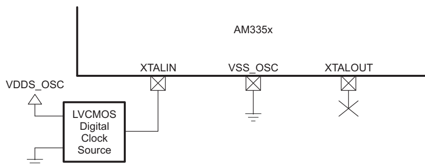
图 6-11. OSC0 LVC MOS 电路原理图
