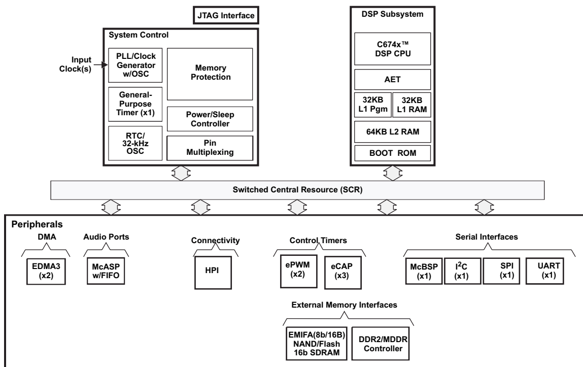
图 1-1. 功能方框图
