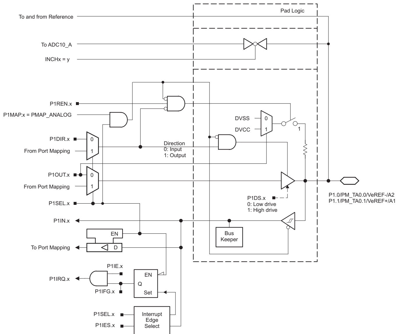
图 6-4. Port P1 (P1.0 and P1.1) Diagram
