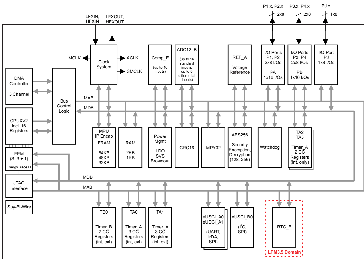
图 1-1. 功能方框图
