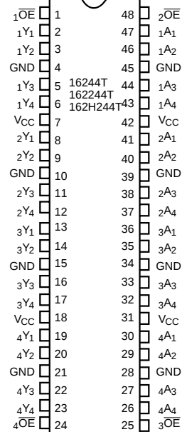
FCT16244-5
