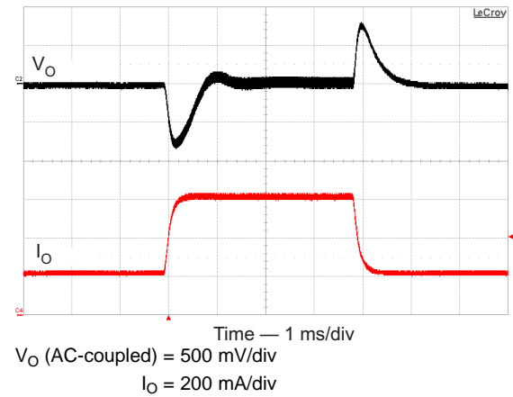
图 20. Load Transient Response
