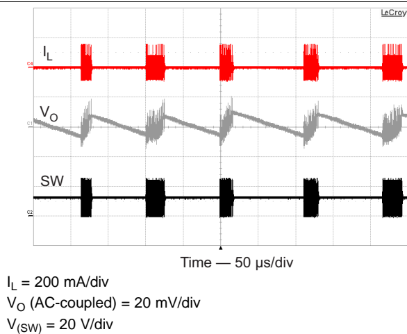
图 23. Pulse Skipping
