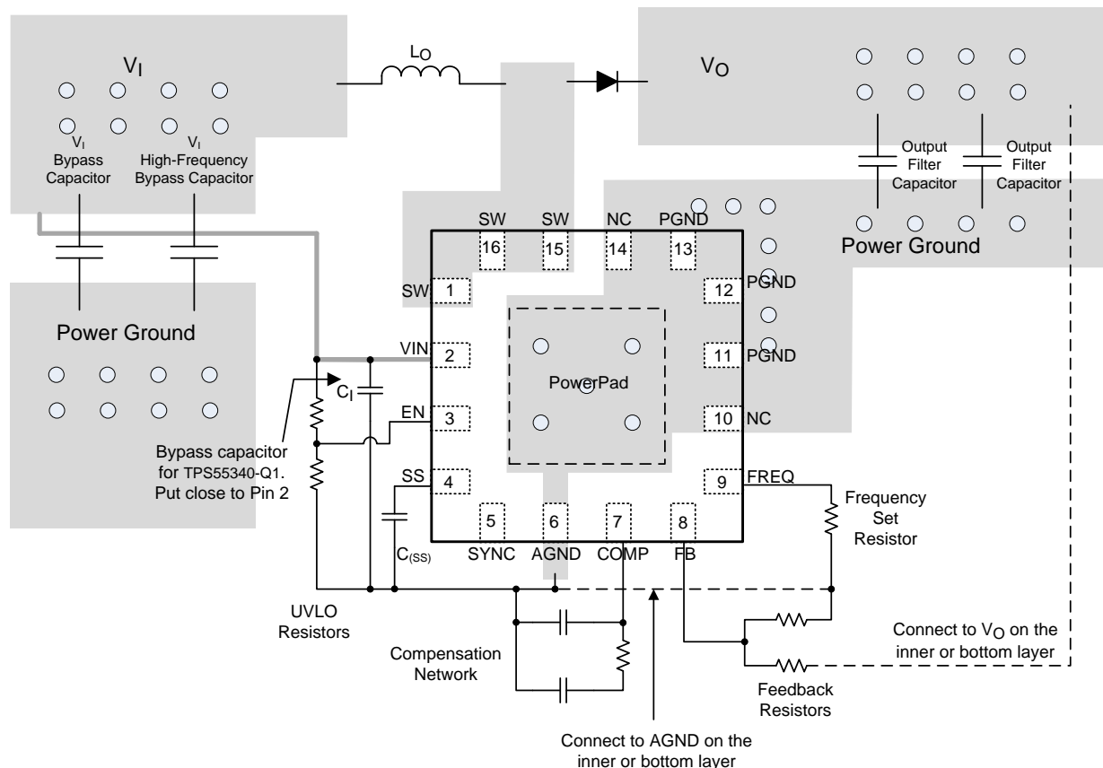
图 33. TPS55340-Q1 Example Board Layout
