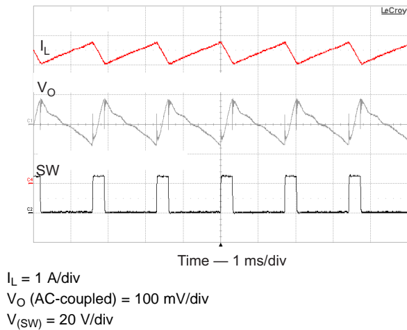
图 21. CCM PWM Operation
