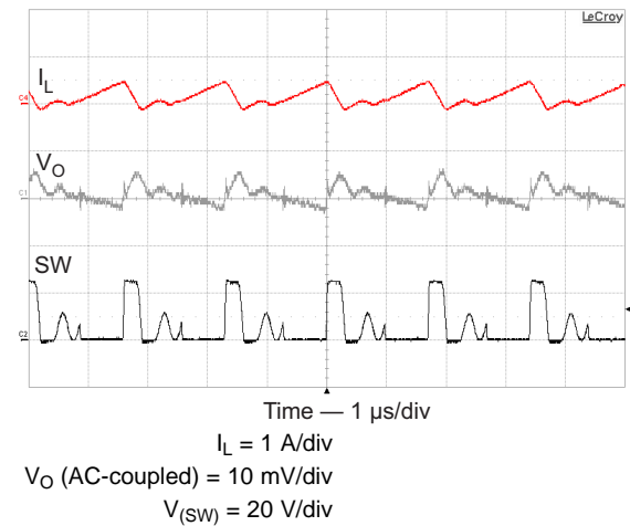
图 22. DCM PWM operation
