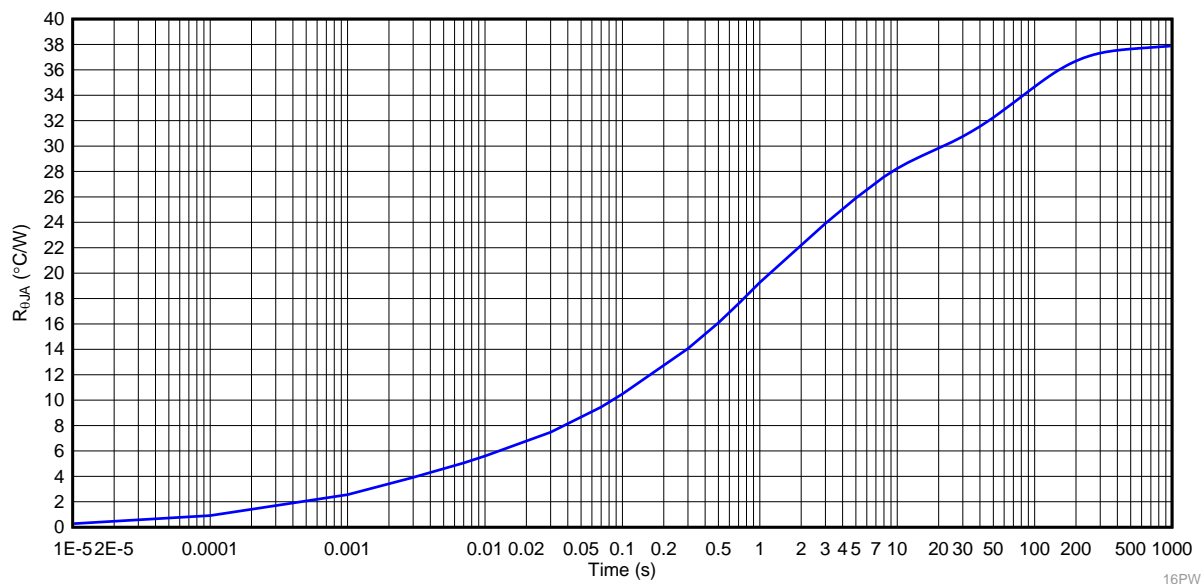
图 16. TPS1HB50-Q1 Transient Thermal Impedance
