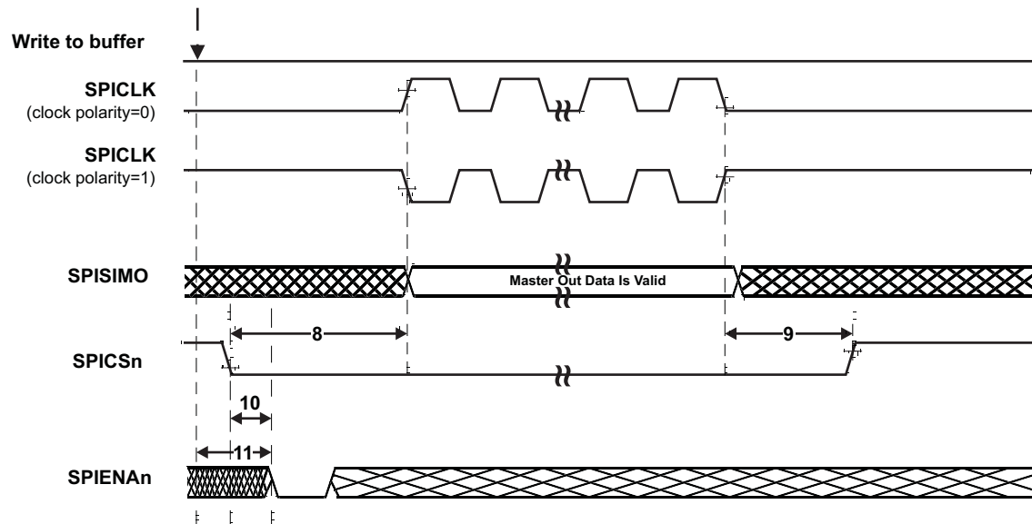
图 5-9. SPI 主控模式芯片选择时序 (时钟相位 = 1)
