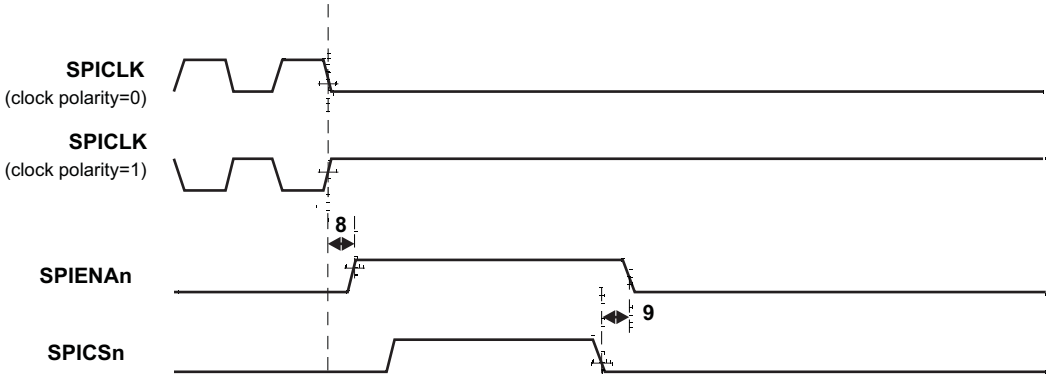
图 5-11. SPI 受控模式使能时序（时钟相位 = 0）
