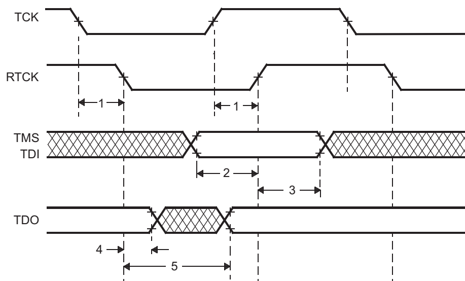
图 6-28. JTAG Timing
