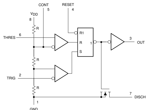
简化原理图
