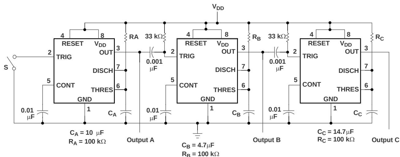
图 18. 顺序计时器电路
