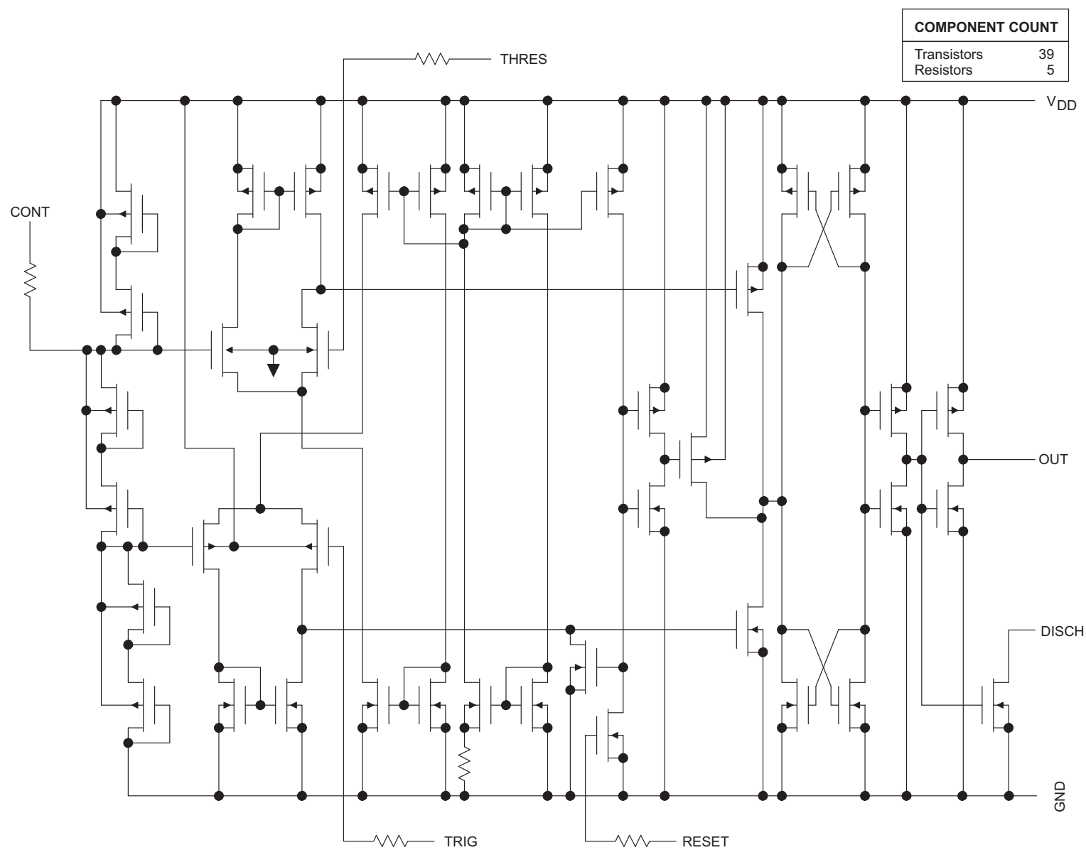
图 11. 等效原理图
