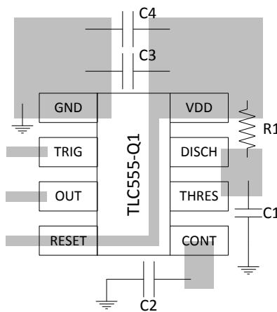
图 20. 建议布局
