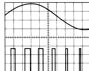
脉宽调制器波形： 上面的波形 - 调制 下面的波形 - 输出电压
